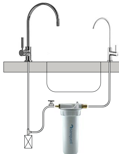
Anschlussschema mit separatem Auslaufhahn
